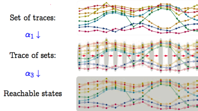
Figura 38: Astrazione degli stati raggiungibili ( \alpha_3 ): dalle tracce concrete all'insieme globale degli stati visitati.
