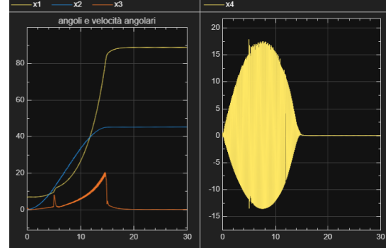
Figure 42: Dinamica degli stati utilizzando un controllo ottimo con PID sul sistema non lineare su cui agisce il disturbo a gradino per t=5s
