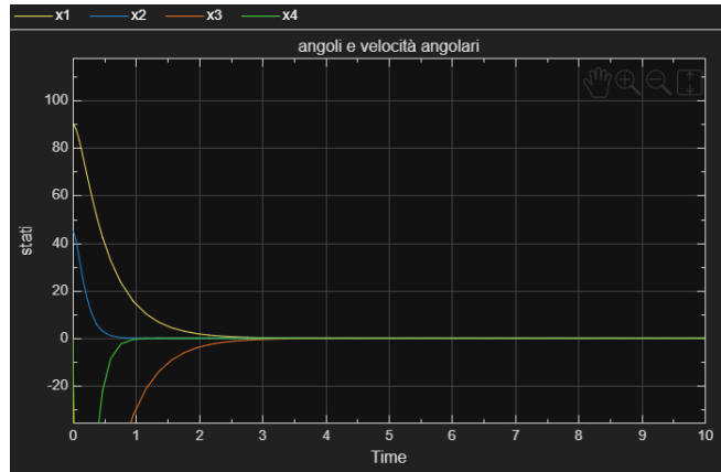
Figure 10: Risultati controllo stabilizzante su sistema linearizzato
