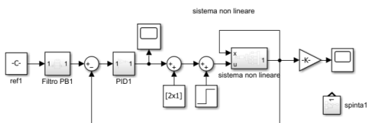
Figure 19: Schema Simulink controllo PID su sistema non lineare con disturbo a gradino sull'ingresso
