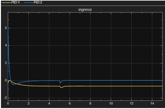
Figure 26: Ingressi utilizzando PID nel sistema linearizzato con disturbo a "spinta"
