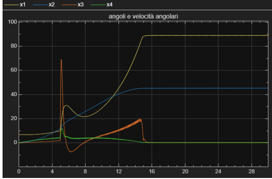
Figure 41: Dinamica degli stati utilizzando un controllo ottimo con PID sul sistema linearizzato su cui agisce il disturbo a gradino per t=5s
