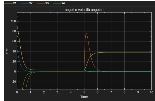
Figure 16: Risultati controllo stabilizzante con disturbo a gradino in ingresso su sistema non lineare
