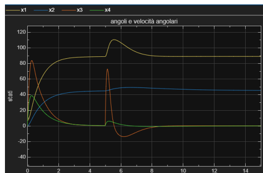
Figure 18: Risultati controllo PID su sistema linearizzato con disturbo a gradino sull'ingresso
