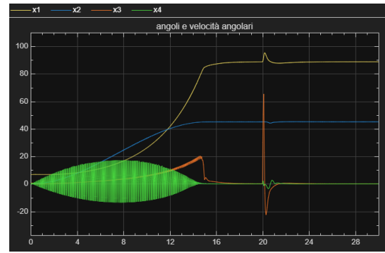
Figure 38: Dinamica degli stati utilizzando un controllo ottimo con PID sul sistema non lineare su cui agisce il disturbo a spinta
