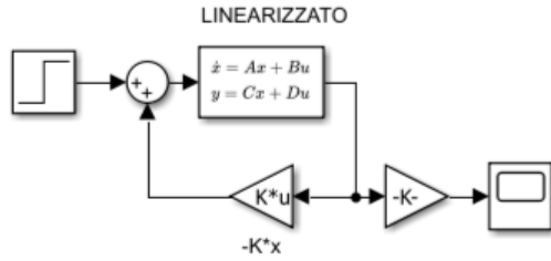
Figure 13: Schema Simulink controllore stabilizzante con disturbo a gradino in ingresso su sistema linearizzato
