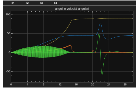
Figure 34: Dinamica degli stati utilizzando un controllo ottimo con PID sul sistema non lineare su cui agisce il disturbo a gradino
