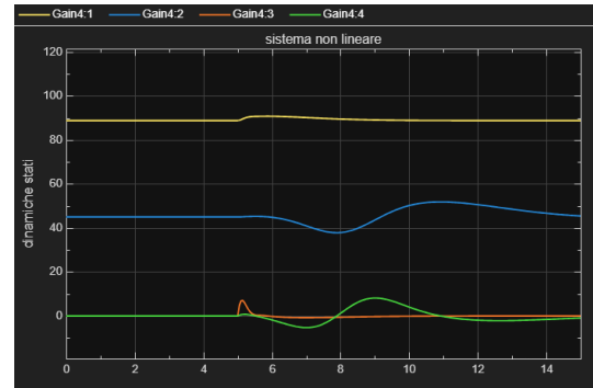
Figure 48: Risultati controllo MPC su sistema non lineare con disturbo a gradino sull'ingresso
