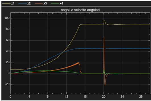
Figure 37: Dinamica degli stati utilizzando un controllo ottimo con PID sul sistema linearizzato su cui agisce il disturbo a spinta
