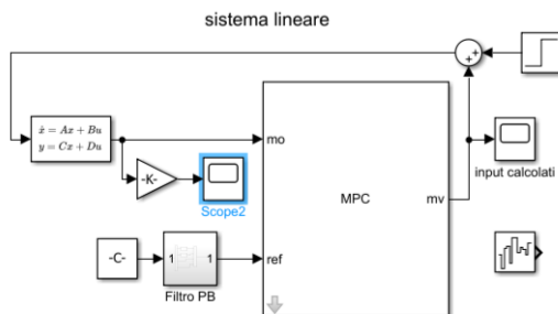
Figure 45: Schema di controllo MPC su sistema linearizzato
