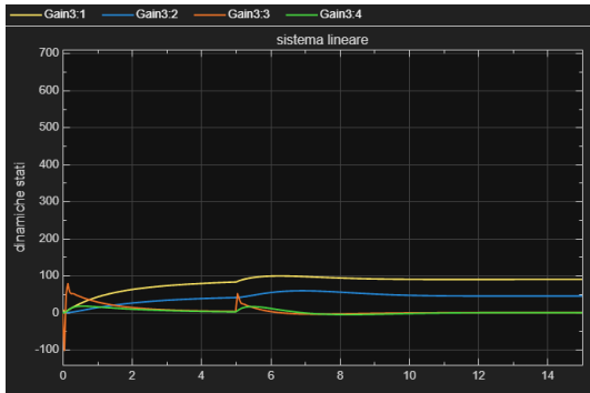
Figure 47: Risultati controllo MPC su sistema linearizzato con disturbo a gradino sull'ingresso
