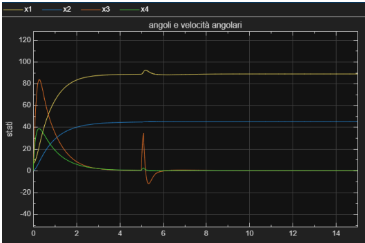
Figure 24: Risultati controllo PID su sistema linearizzato con disturbo a spinta sull'ingresso
