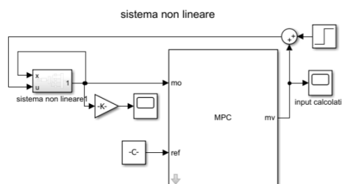
Figure 46: Schema di controllo MPC su sistema non lineare
