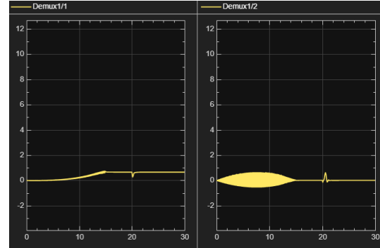
Figure 40: Ingressi generati dal controllo ottimo con PID, agenti sul sistema non lineare su cui agisce il disturbo a spinta
