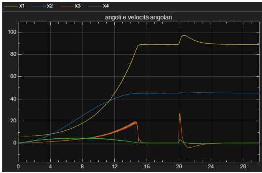
Figure 33: Dinamica degli stati utilizzando un controllo ottimo con PID sul sistema linearizzato su cui agisce il disturbo a gradino
