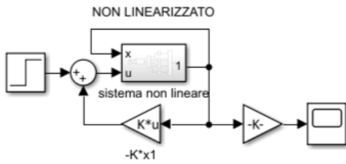
Figure 15: Schema Simulink controllore stabilizzante con disturbo a gradino in ingresso su sistema non lineare
