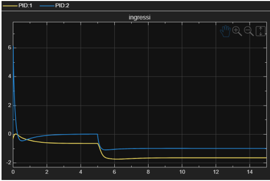
Figure 21: Ingressi utilizzando PID nel sistema linearizzato con disturbo a gradino
