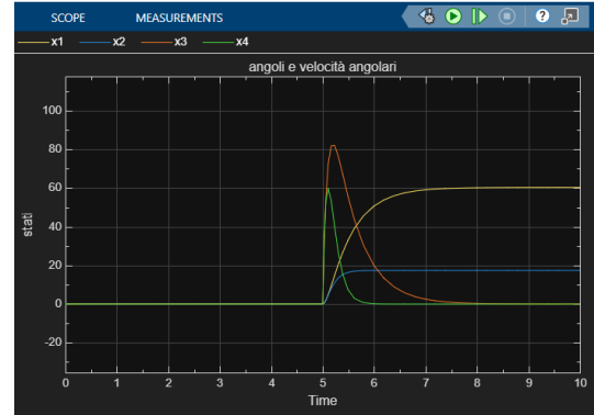
Figure 14: Risultati controllo stabilizzante con disturbo a gradino in ingresso su sistema non lineare
