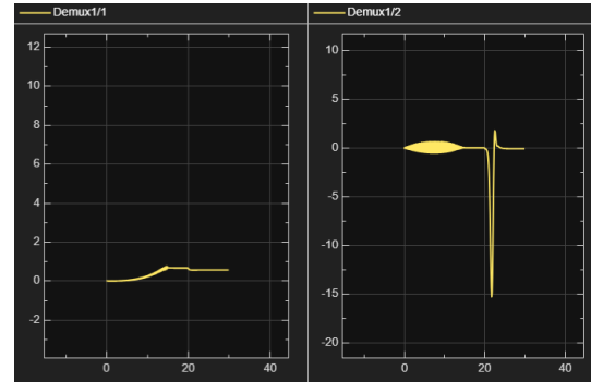
Figure 36: Ingressi generati dal controllo ottimo con PID, agenti sul sistema non lineare su cui agisce il disturbo a gradino
