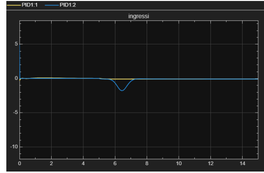
Figure 22: Ingressi utilizzando PID nel sistema non lineare con disturbo a gradino
