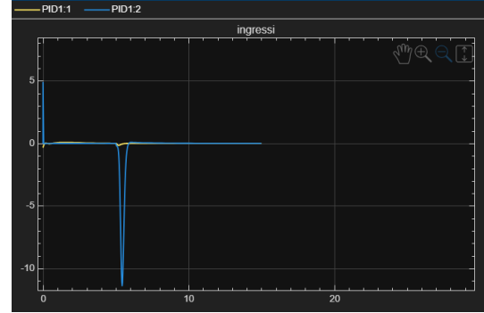
Figure 27: Ingressi utilizzando PID nel sistema non lineare con disturbo a "spinta"
