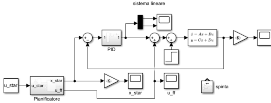
Figure 32: Schema Simulink controllo ottimo con PID
