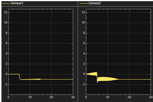
Figure 43: Ingressi generati dal controllo ottimo con PID, agenti sul sistema linearizzato su cui agisce il disturbo a gradino per t=5s
