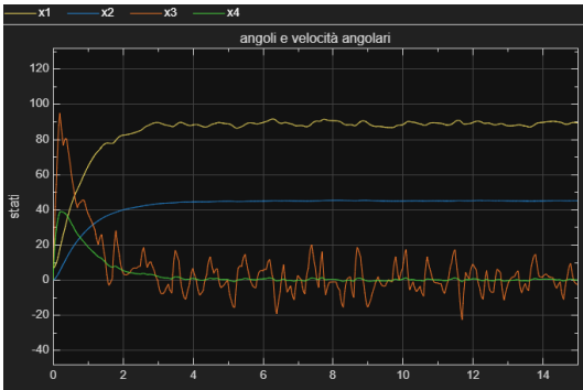
Figure 28: Risultati controllo PID su sistema linearizzato con disturbo White Noise sull'ingresso
