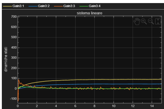
Figure 51: Risultati controllo MPC su sistema linearizzato con disturbo White Noise sull'ingresso
