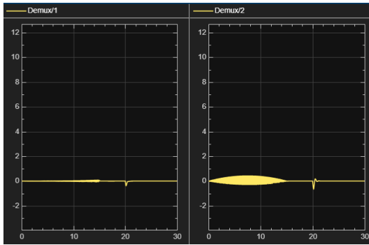
Figure 39: Ingressi generati dal controllo ottimo con PID, agenti sul sistema linearizzato su cui agisce il disturbo a spinta
