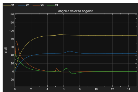
Figure 20: Risultati controllo PID su sistema non lineare con disturbo a gradino sull'ingresso
