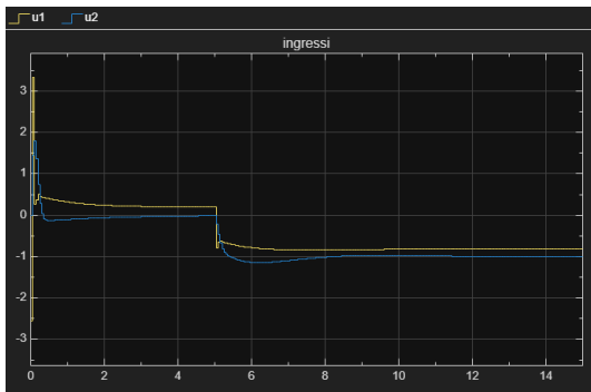
Figure 49: Ingressi di controllo MPC su sistema linearizzato con disturbo a gradino sull'ingresso
