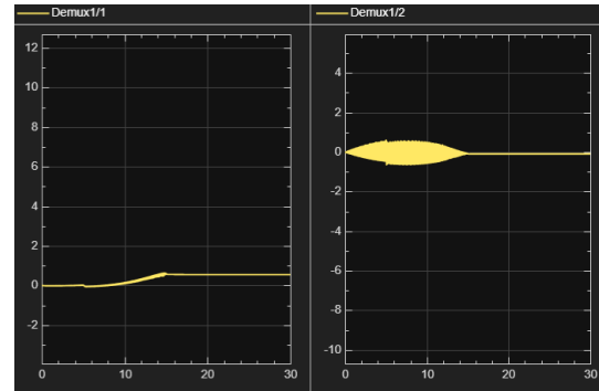
Figure 44: Ingressi generati dal controllo ottimo con PID, agenti sul sistema non lineare su cui agisce il disturbo a gradino per t=5s
