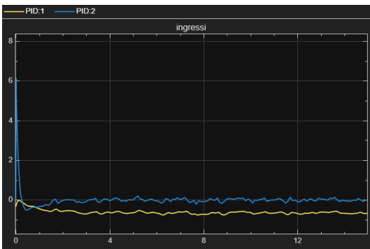
Figure 30: Ingressi utilizzando PID nel sistema linearizzato con disturbo White Noise
