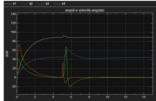
Figure 25: Risultati controllo PID su sistema non lineare con disturbo a spinta sull'ingresso
