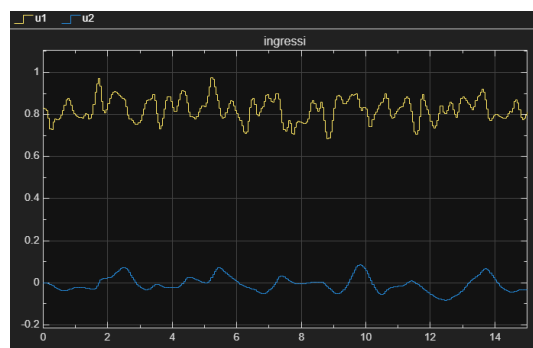
Figure 54: Ingressi di controllo MPC su sistema non lineare con disturbo White Noise sull'ingresso
