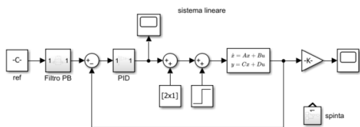
Figure 17: Schema Simulink controllo PID su sistema linearizzato con disturbo sull'ingresso
