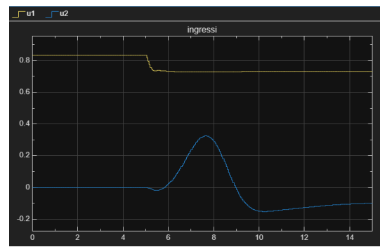
Figure 50: Ingressi di controllo MPC su sistema non lineare con disturbo a gradino sull'ingresso
