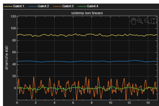
Figure 52: Risultati controllo MPC su sistema non lineare con disturbo White Noise sull'ingresso
