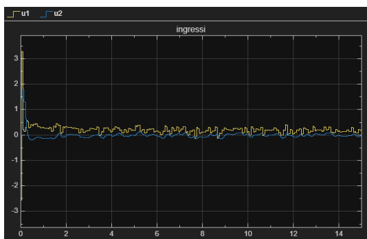
Figure 53: Ingressi di controllo MPC su sistema linearizzato con disturbo White Noise sull'ingresso
