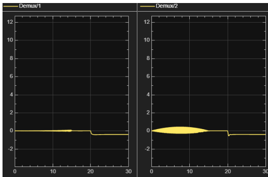
Figure 35: Ingressi generati dal controllo ottimo con PID, agenti sul sistema linearizzato su cui agisce il disturbo a gradino
