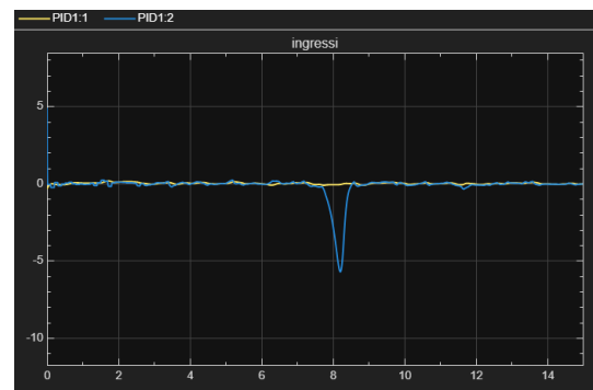
Figure 31: Ingressi utilizzando PID nel sistema non lineare con disturbo White Noise
