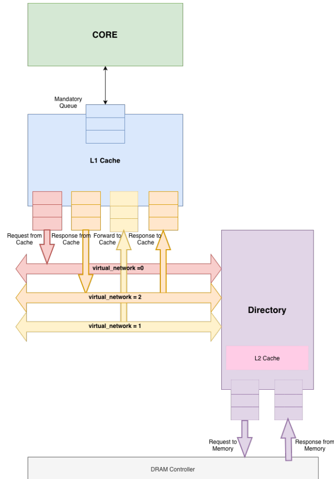
Figura 2.7: Schema d'interconnessioni della Directory
