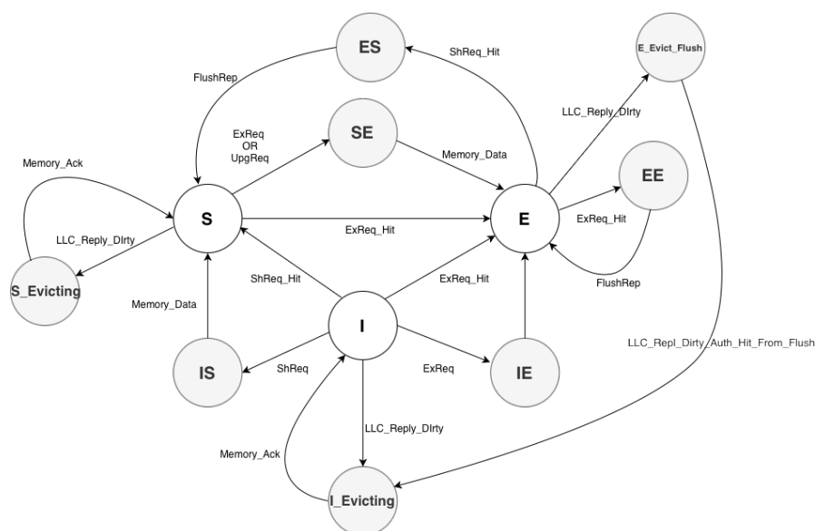
Figura 2.3: Automa a stati finiti per i Data Chunk
