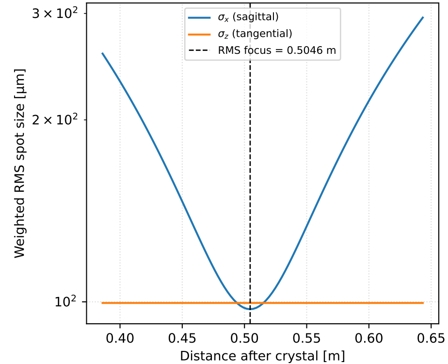
Longitudinal focal scan
