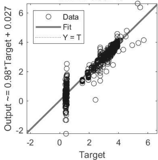
All: R=0.99246
