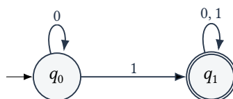
Figura 1.2. Automa che riconosce le parole contenenti almeno un uno
