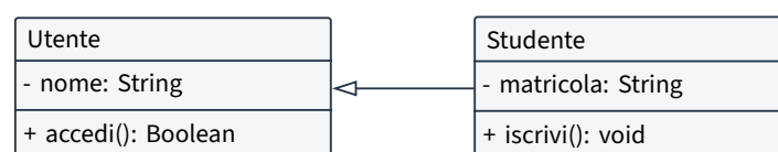
Figura 1.6. Diagramma UML delle classi utente e studente
