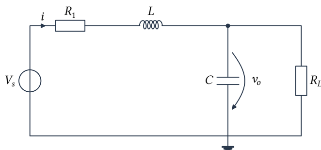
Figura 1.3. Filtro RLC del secondo ordine con carico resistivo
