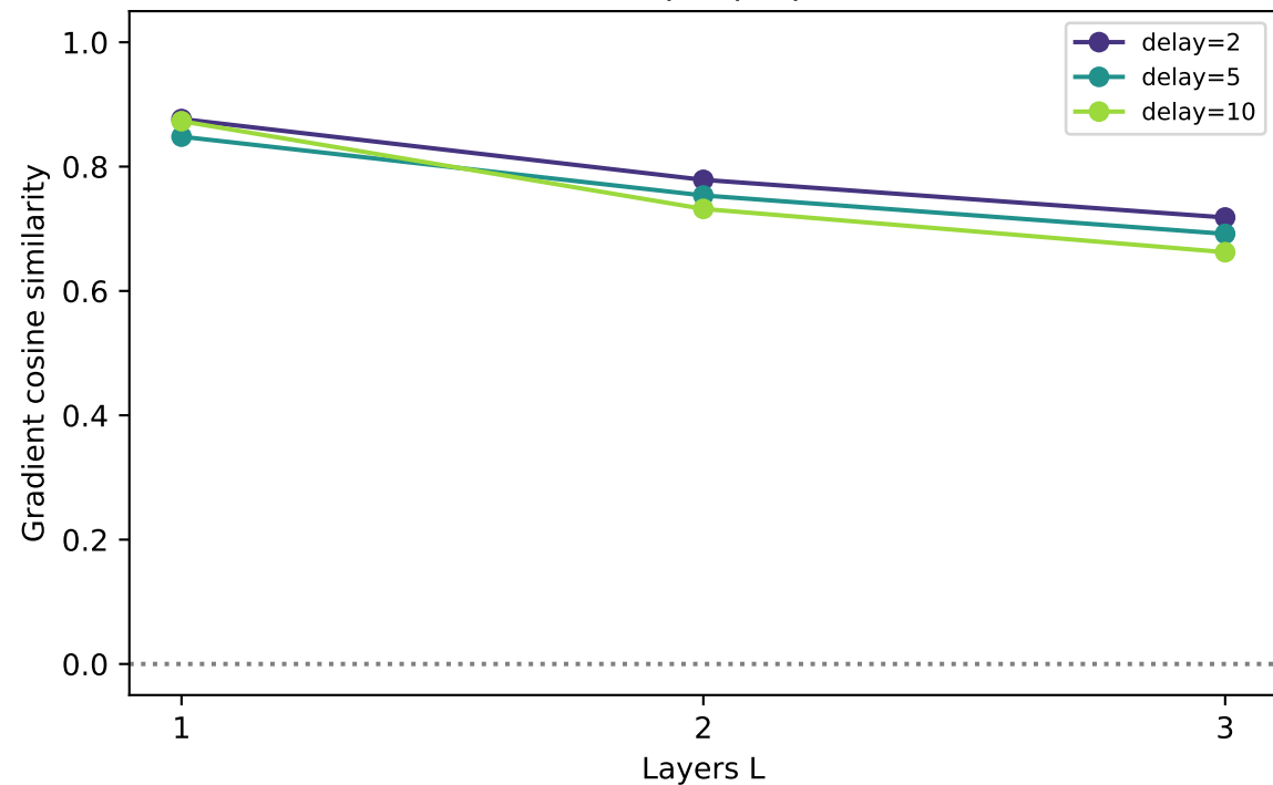
Deep e-prop
