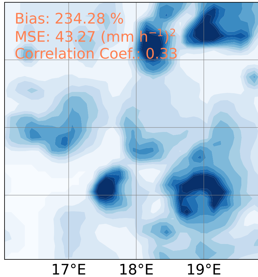
(b) IMERG (IR)
