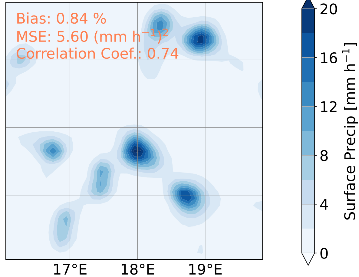
(c) GPROF-IR (GMI, 3)
