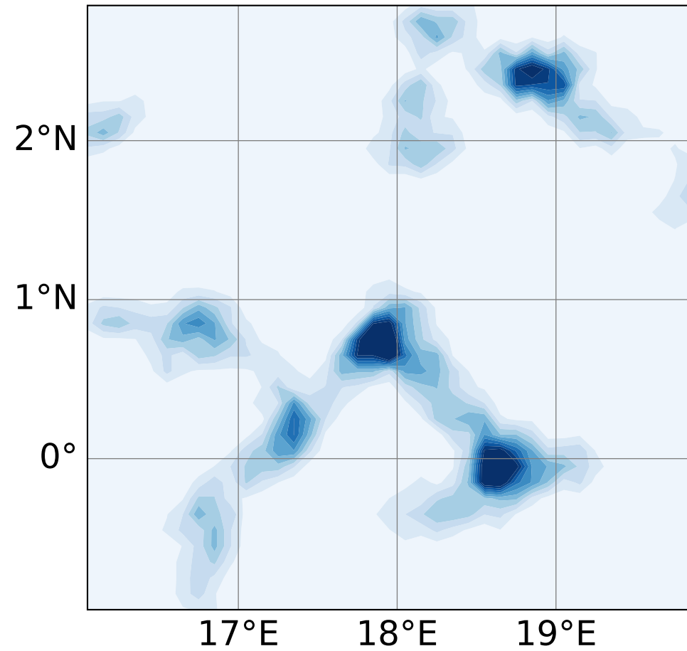
(a) GPROF V08 (SSMIS)
