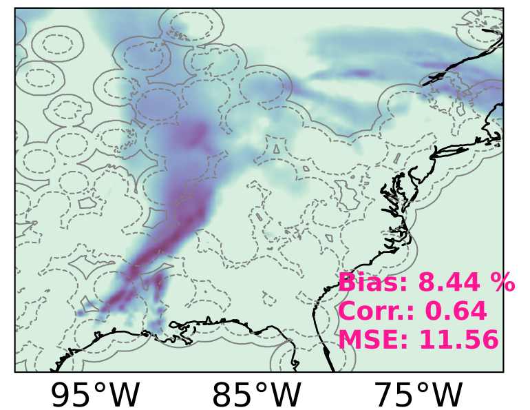
(g) GPROF IR (GMI, 3)
