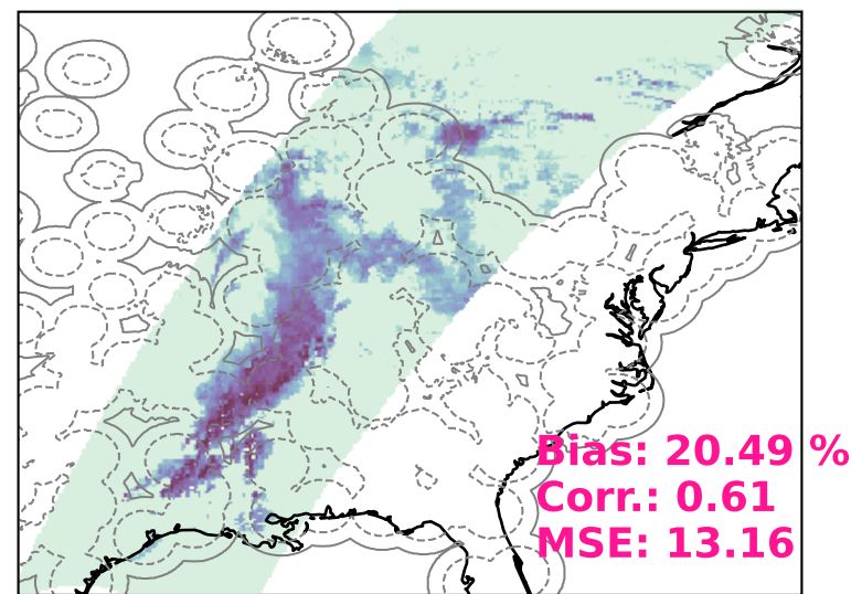
(f) GPROF IR (GMI)
