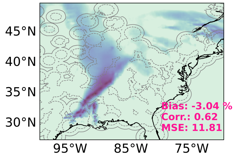
(e) GPROF IR (CMB)
