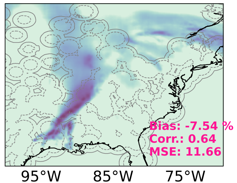
(f) GPROF IR (GMI)
