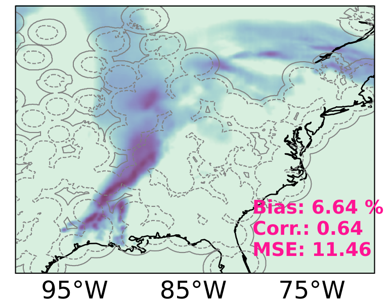
(h) GPROF IR (GMI, 5)
