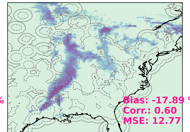
(h) GPROF IR (GMI, 5)
