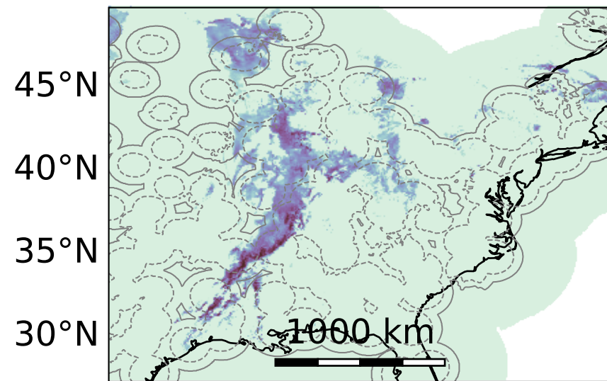
(e) GPROF IR (CMB)
