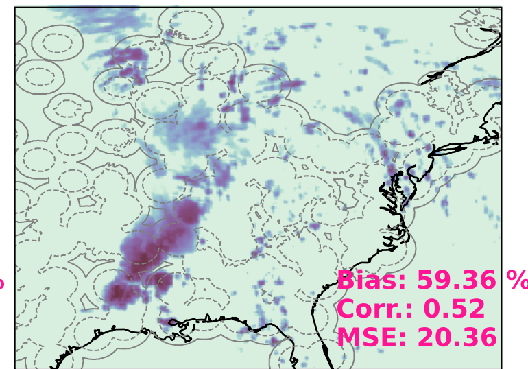
(g) GPROF IR (GMI, 3)
