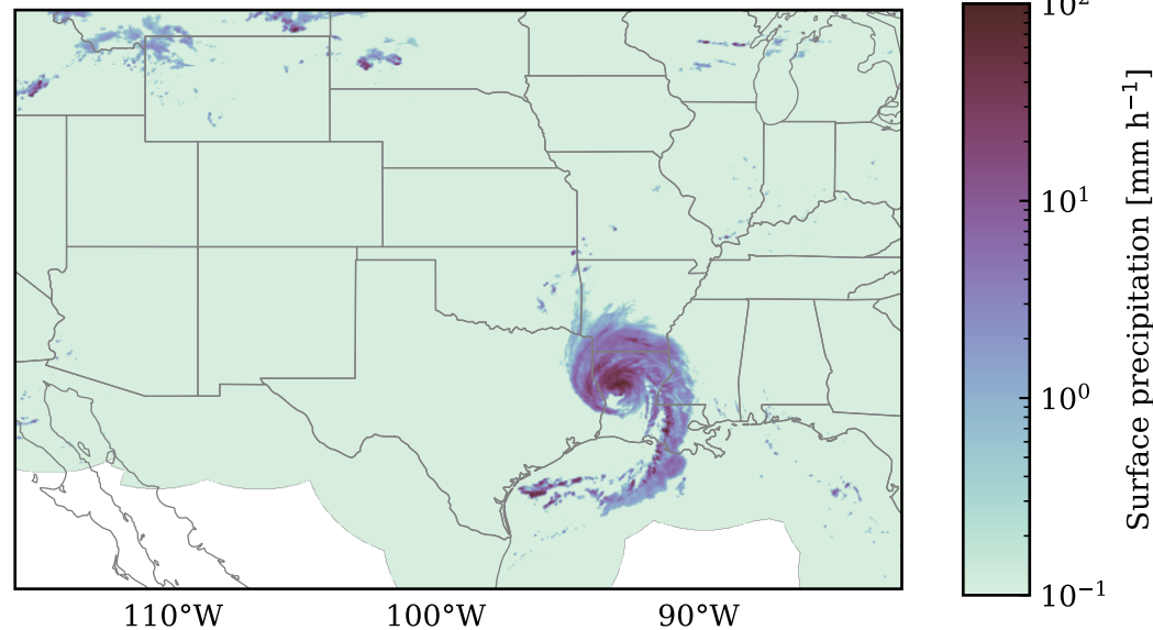
(d) Surface precipitation
