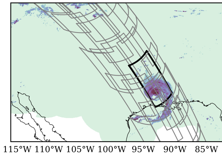
(d) MRMS surface precipitation
