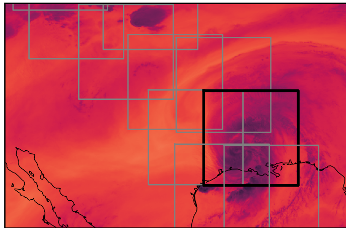
(d) MRMS surface precipitation
