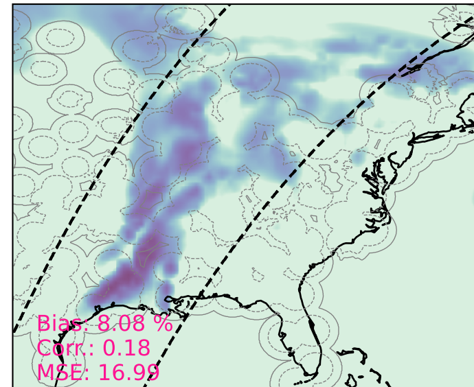
(b) ERA5
