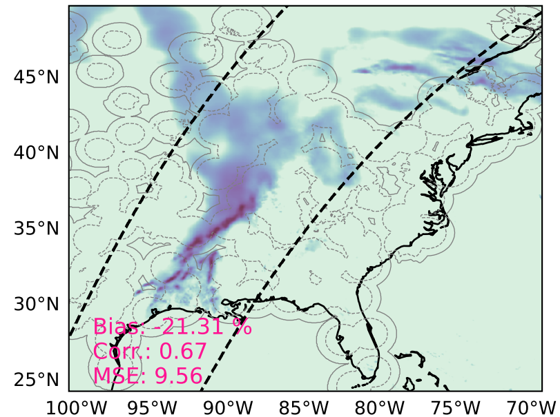
(d) SatRain (Geo IR)
