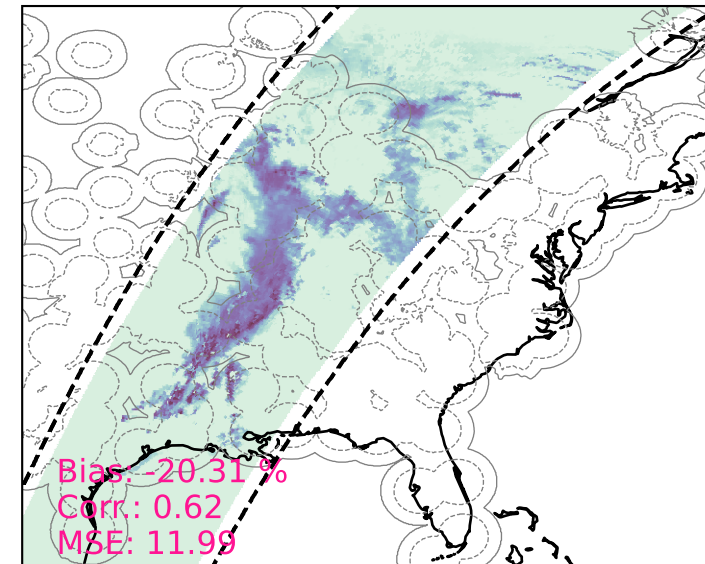
(c) GPROF V7 (GMI)
