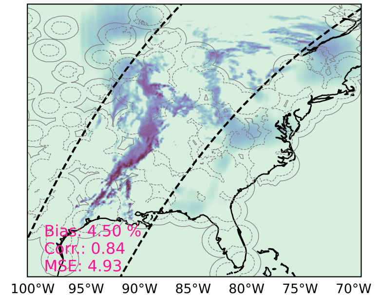
(f) SatRain (GMI)
