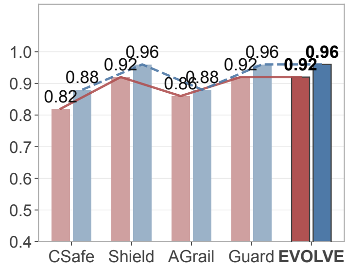
Multilingual
