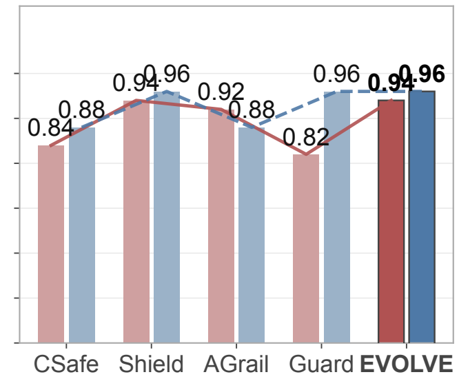
PAP
