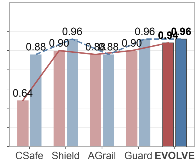
ReneLLM
