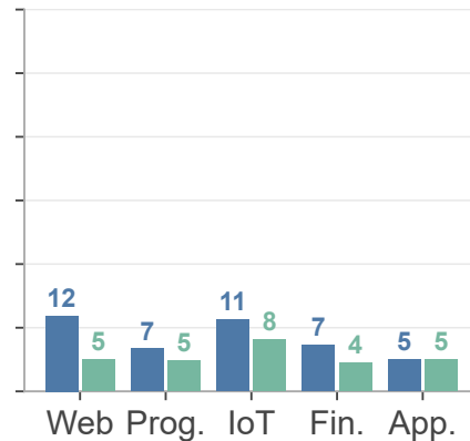
Claude
