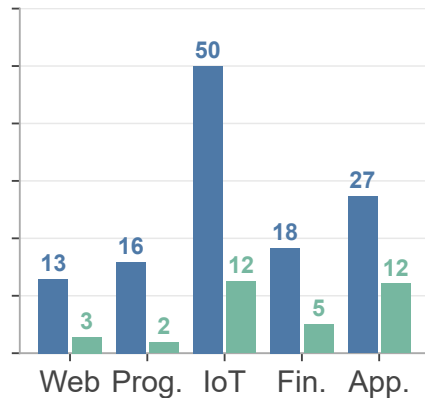
GPT-4o
