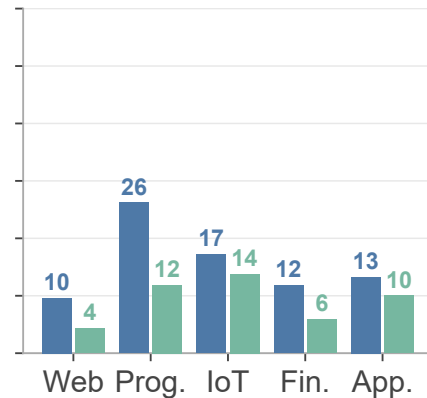
Gemini
