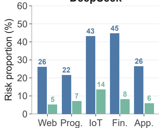
DeepSeek
