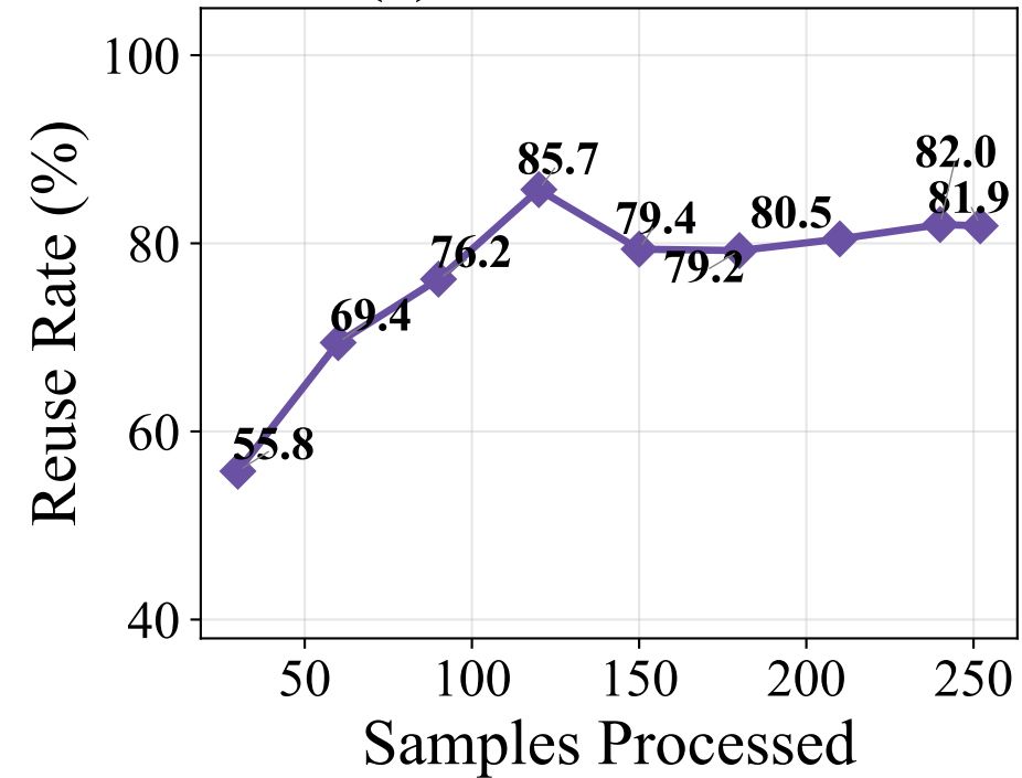
(d) Tool Reuse Rate
