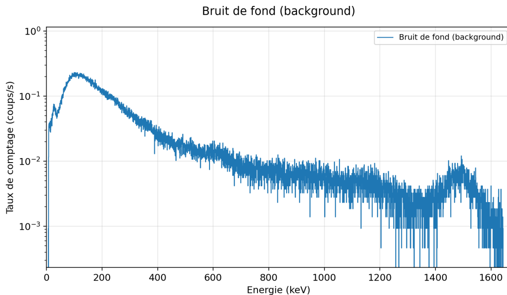
FIGURE 1 – Spectre de fond (background), généré par le code Python dans le dossier scripts (chemin relatif remontant d'un niveau depuis le dossier rapport ).
