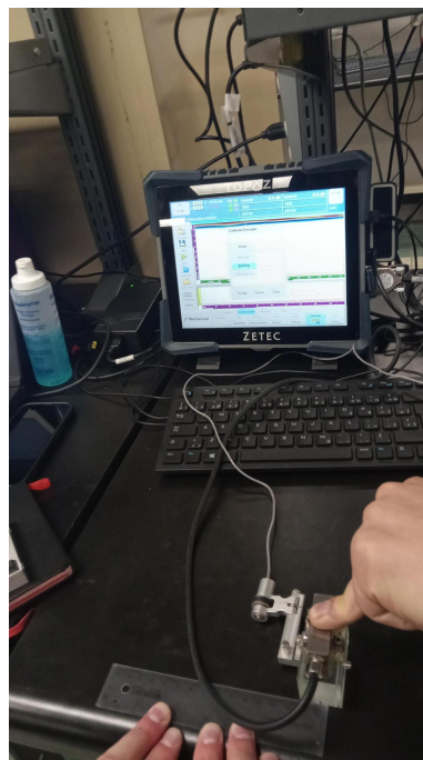
FIGURE 12 – Calibration de l'encodeur.
