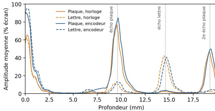
FIGURE 2 – A-scans moyens sur la plaque (traits pleins) et sous les lettres (tirets), sans encodeur (orange) et avec encodeur (bleu). Les lignes pointillées grises marquent la position moyenne de chaque écho dans les deux acquisitions.
