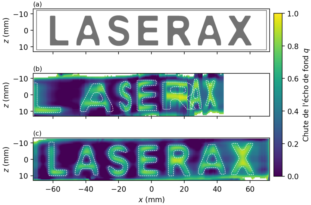
FIGURE 3 – Lettres du CAD (a) et chute de l'écho de fond q sans encodeur (b) et avec encodeur (c). Le pointillé blanc est le contour CAD de chaque lettre, placé sur la mesure avec son propre décalage et son propre étirement.
