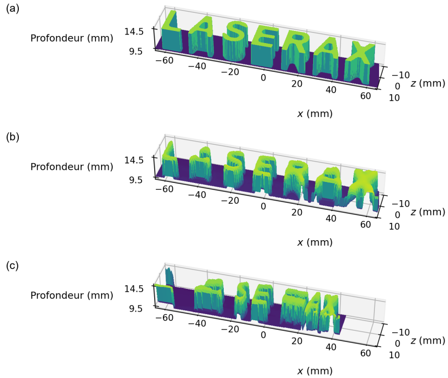
FIGURE 4 – Surface du CAD (a) et surfaces reconstruites avec encodeur (b) et sans encodeur (c), avec le pas nominal de 0,25 mm. L'axe vertical est la profondeur de l'écho le plus profond, exagérée trois fois.
