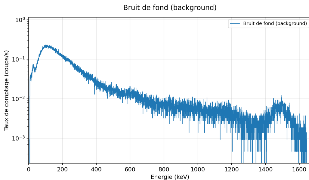
FIGURE 1 – Spectre de fond (background), généré par le code Python dans le dossier Analyse (chemin relatif remontant d'un niveau depuis le dossier Rapport).
