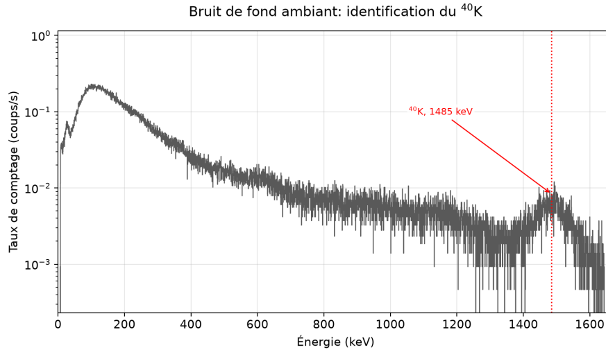
FIGURE 4 – Spectre du bruit de fond ambiant (échelle logarithmique, 36 minutes d'acquisition). La raie identifiée à 1485 \pm 3 \text{ keV} est attribuée au ^{40}\text{K} (1460,8 keV), présent naturellement dans le béton, la brique et le corps humain.
