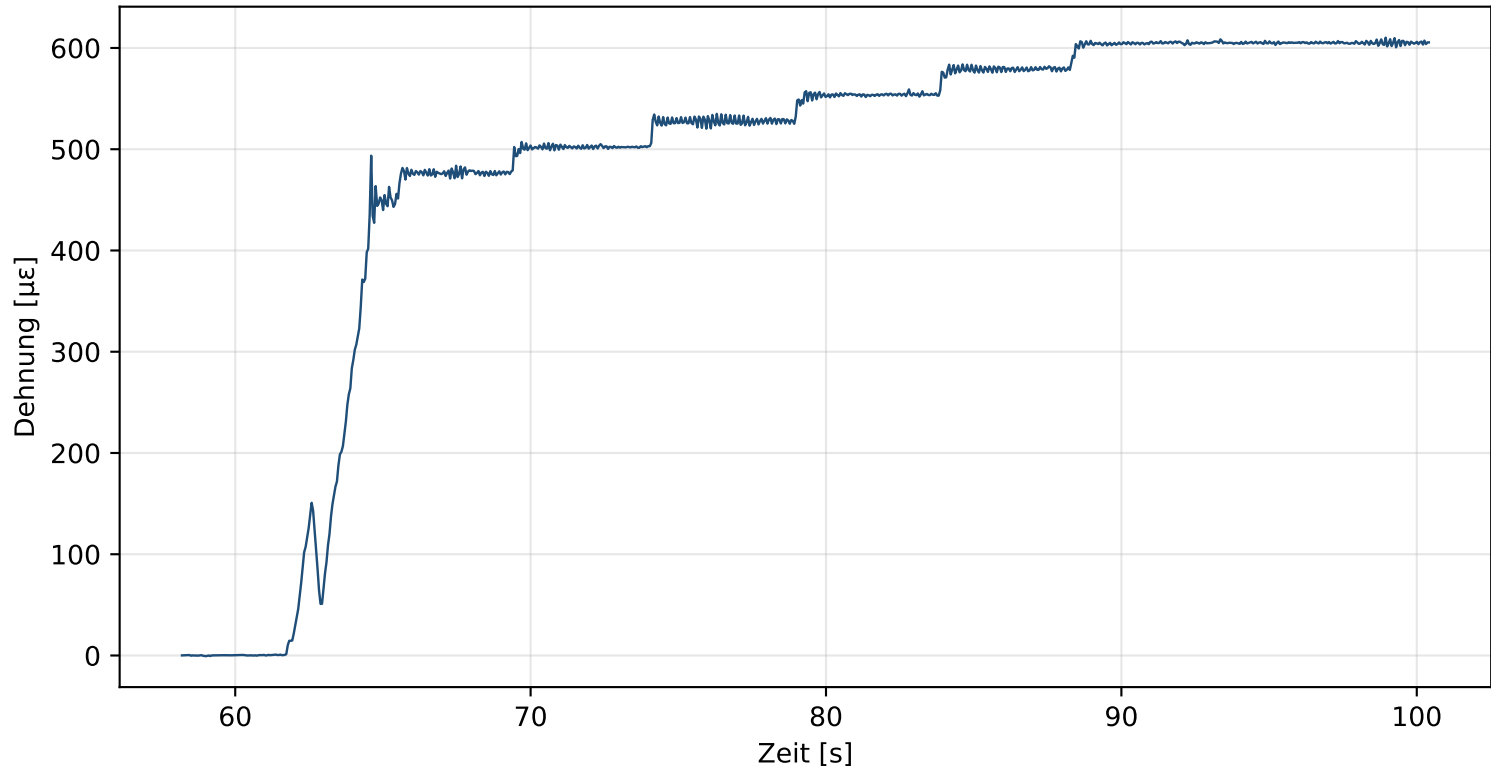
DMS-Messung - Gewichtsbelastung (Viertelbrücke)
