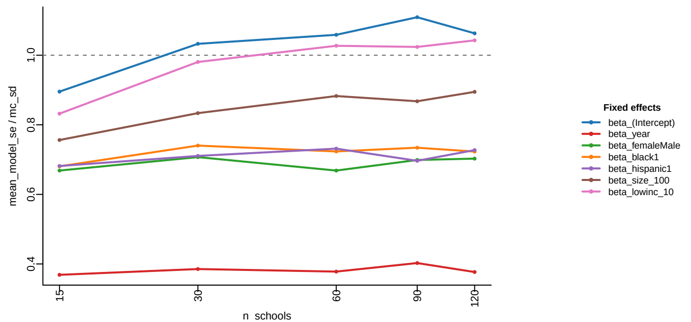
Model B : Fixed-Effect SE Calibration
