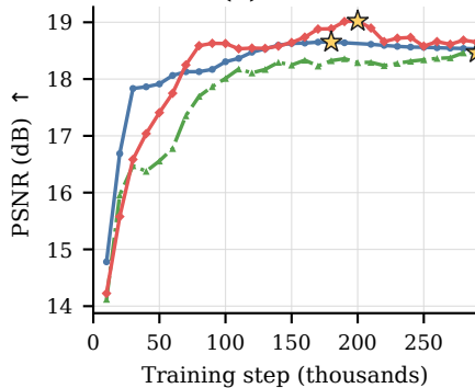
(b) PSNR
