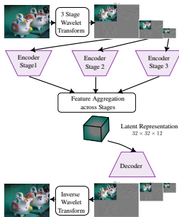
LiteVAE
