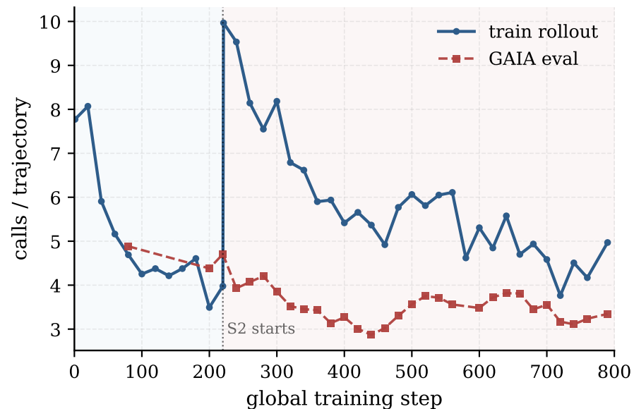
(d) Search-tool calls
