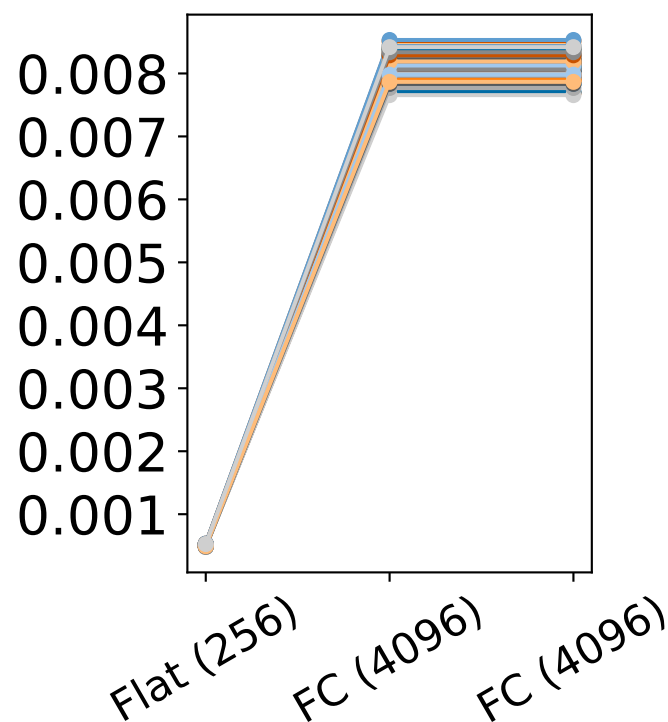
AlexNet-CIFAR-100
