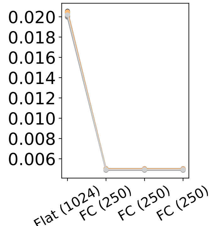
CNN-CIFAR-10
