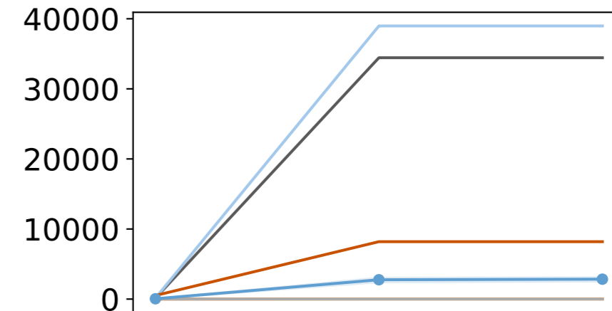
AlexNet-CIFAR-100
