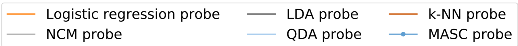
MLP-MNIST
