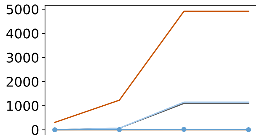
MLP-MNIST
