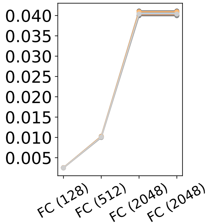
AlexNet-CIFAR-100
