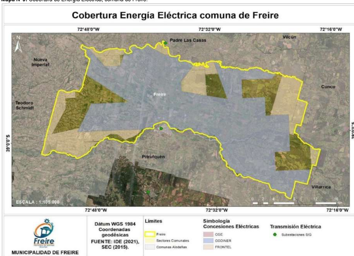
Mapa N°9: Cobertura de Energía Eléctrica, comuna de Freire.
