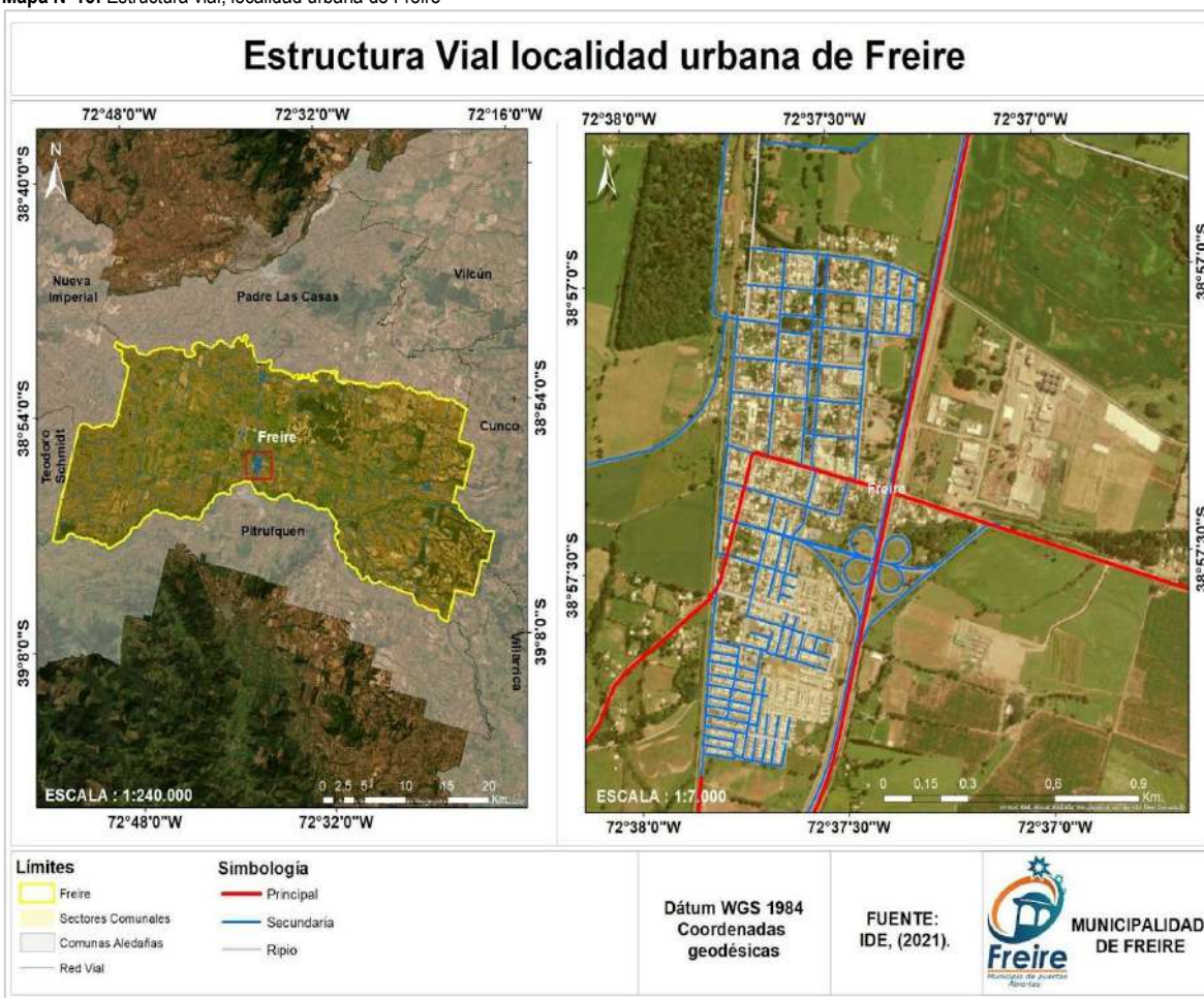
Mapa N°15: Estructura vial, localidad urbana de Freire
