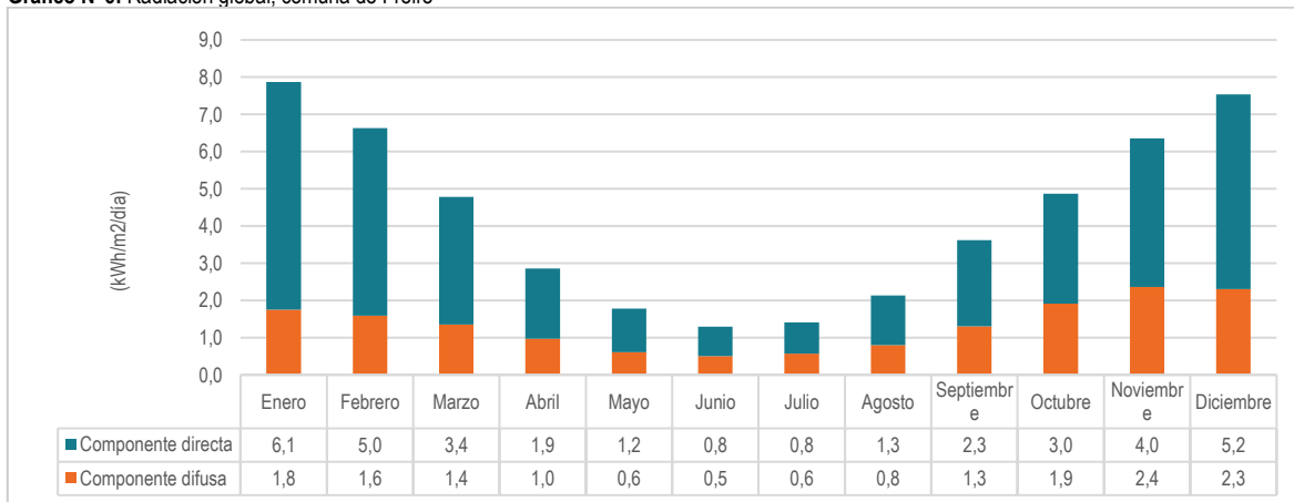
Gráfico N°6: Radiación global, comuna de Freire
