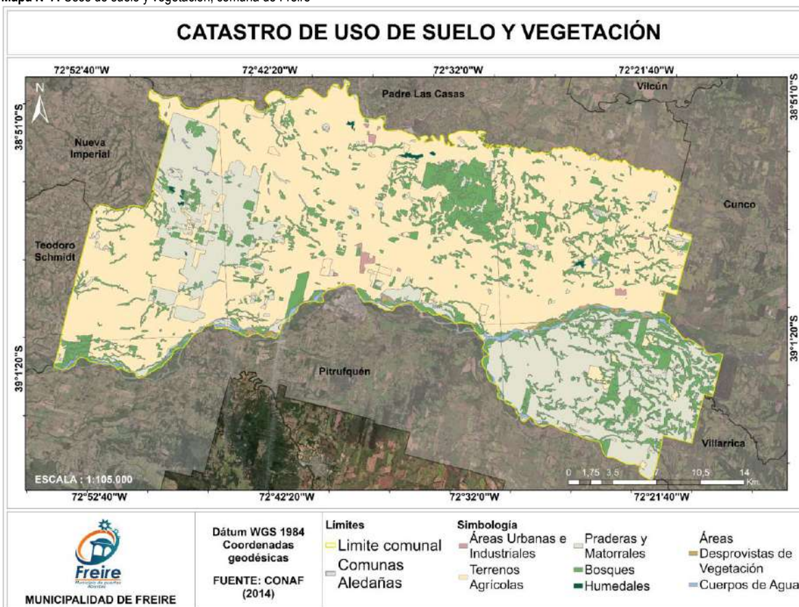
Mapa N°7: Usos de suelo y vegetación, comuna de Freire
