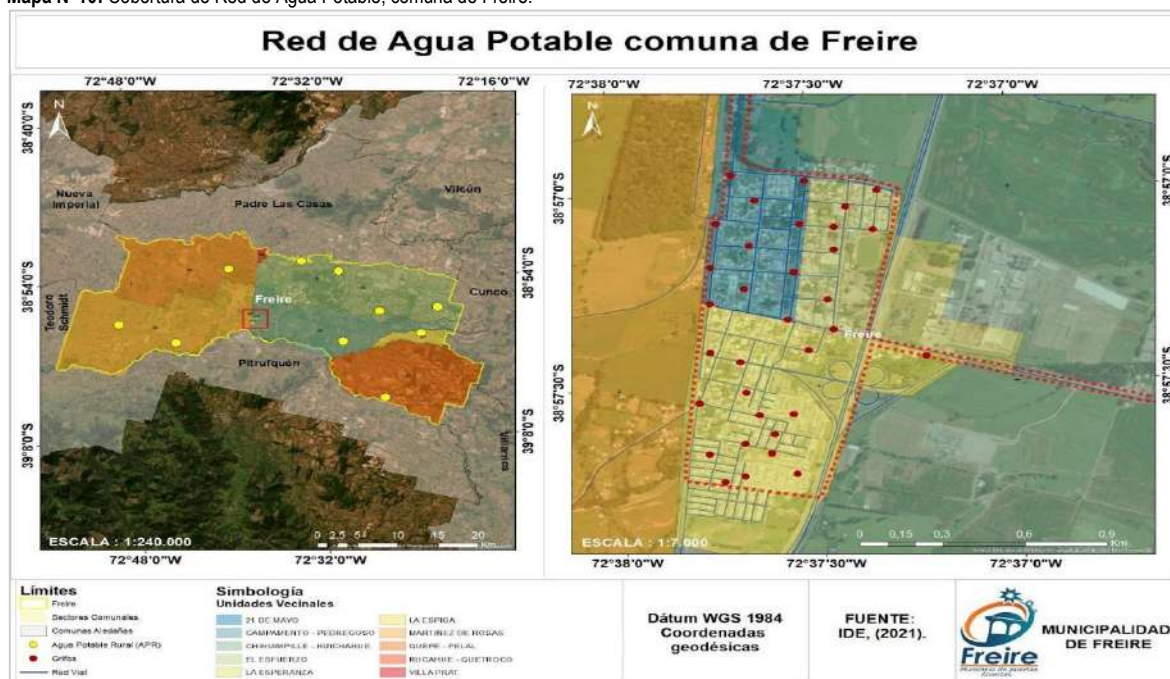
Mapa N°10: Cobertura de Red de Agua Potable, comuna de Freire.
