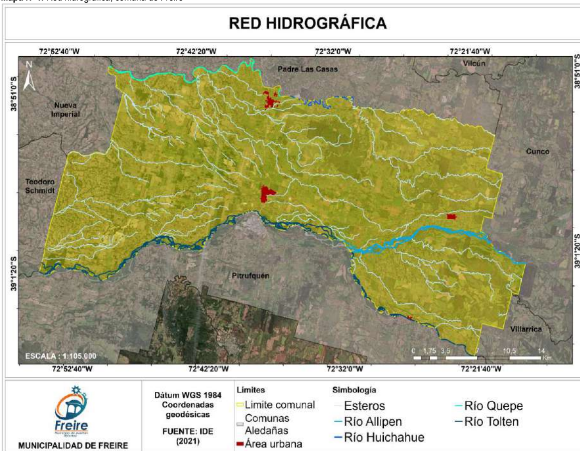
Mapa N°4: Red hidrográfica, comuna de Freire
