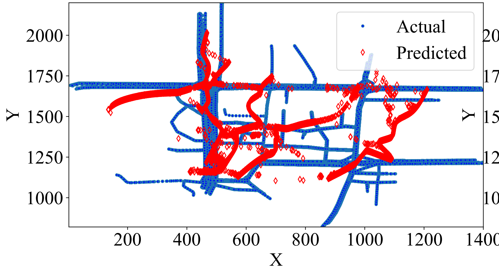
Actual vs Predicted - RNN
