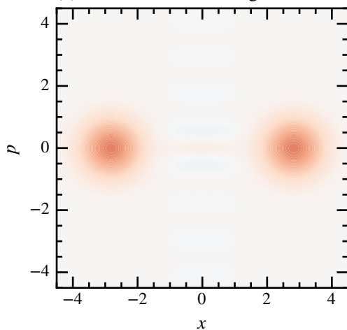
(d) Reduced oscillator Wigner function
