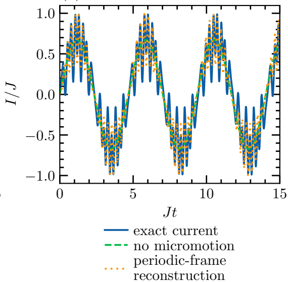
(d) Micromotion-sensitive current
