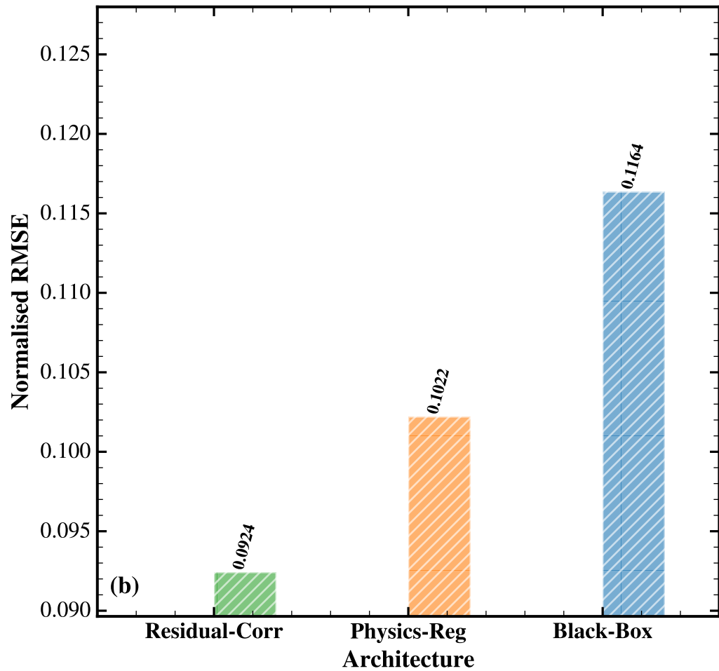
(b) NRMSE
