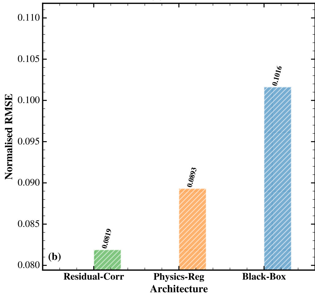
(b) NRMSE
