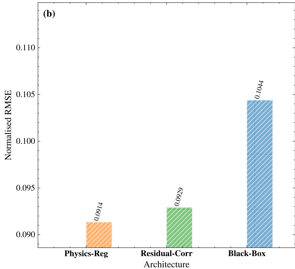
(b) NRMSE
