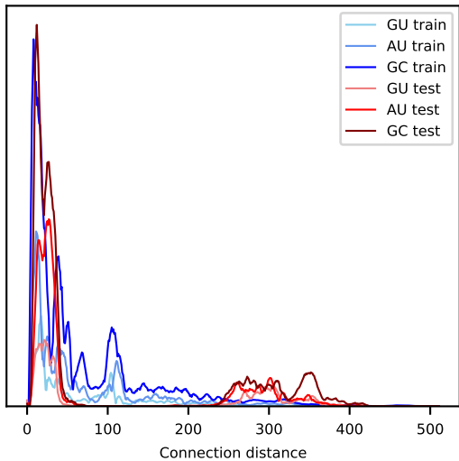
tmRNA
