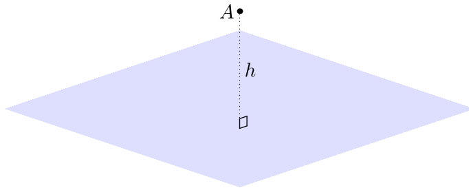
Figure 7: Den korteste avstanden h mellom punktet A og planet (i blått).
