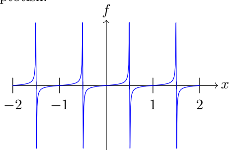
Figure 14: Grafen til f(x) = \tan(\pi x) på intervallet x \in [-2, 2] .
