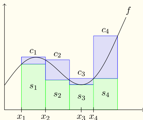
Figur 5.6: Arealene av s_i markert som grønne søyler og arealene av c_i markert som blå søyler. Bredden til hver søyle er \Delta x = \frac{b-a}{n} (her er n = 4 ).
