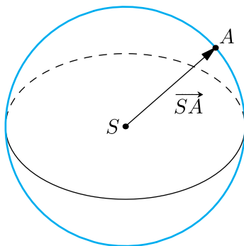
Figure 4: Kule med sentrum S = (x_0, y_0, z_0) . Punktet A = (x, y, z) ligger på kula.
