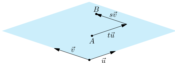
Figur 4.1: Utklipp av planet \alpha utspent av vektorene \vec{v} og \vec{u} .
