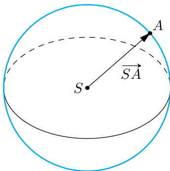
Figur 4.4: Kule med sentrum S = (x_0, y_0, z_0) . Punktet A = (x, y, z) ligger på kula.
