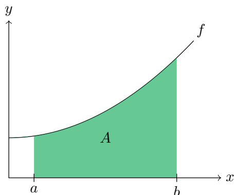
Figur 5.1: Arealet A avgrenset av grafen til f , x -aksen og linjene x = a og x = b .
