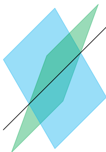
Figur 4.3: Skjæringslinje mellom to plan.
