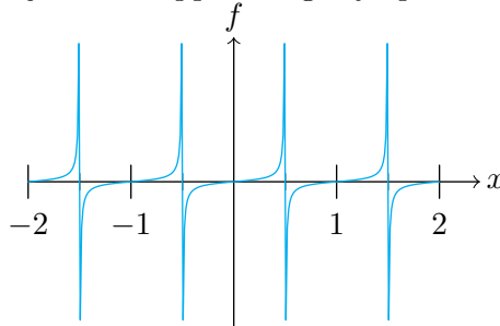
Figur 2.13: Grafen til f(x) = \tan(\pi x) på intervallet x \in [-2, 2] .
