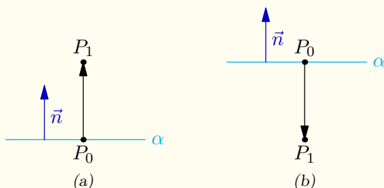
Figur 4.7: a) Vektoren mellom P_0 og P_1 har samme retning som \vec{n} . b) Vektoren mellom P_0 og P_1 har motsatt retning som \vec{n} .
