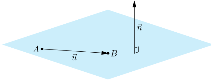
Figur 4.2: Punktene A = (x_0, y_0, z_0) og B = (x, y, z) i planet \alpha med normalvektor \vec{n} = [a, b, c] .
