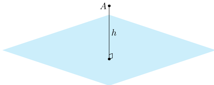
Figur 4.6: Den korteste avstanden h mellom punktet A og planet (i blått).
