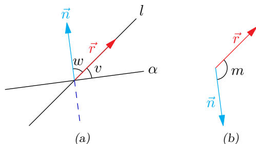
Figur 4.10: a) \vec{n} og \vec{r} utspenner vinkelen w < 90^\circ . b) \vec{n} og \vec{r} utspenner vinkelen m > 90^\circ .
