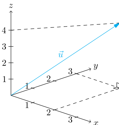
Figur 3.1: Den tredimensjonale vektoren \vec{u} = [2, 3, 4]
