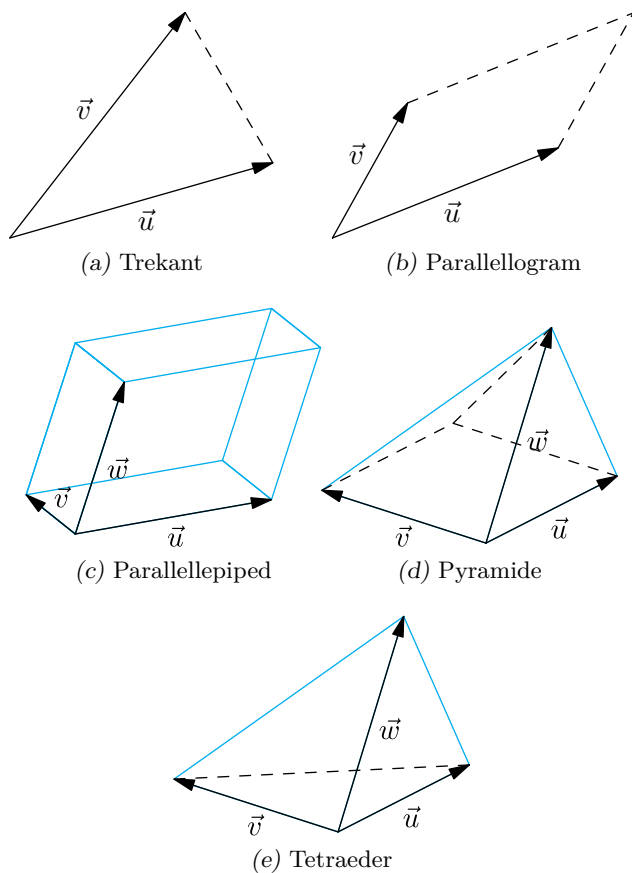
Figur 3.3: Geometriske former utspent av vektorene \vec{u} , \vec{v} og \vec{w} .
