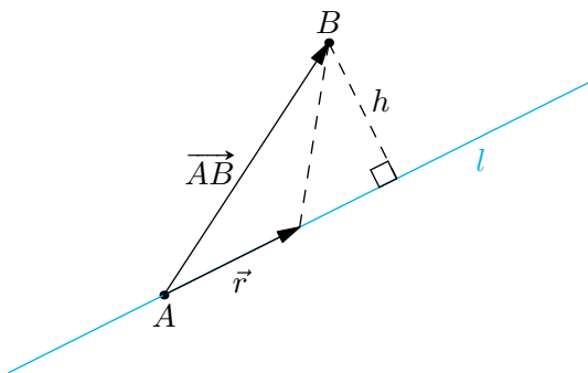
Figur 4.5: Punkt B en avstand h fra linja l .
