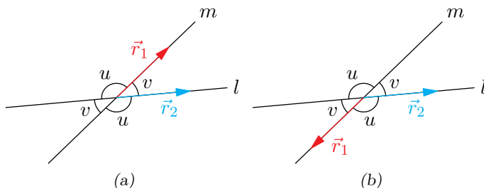
Figur 4.8: a) \vec{r}_1 og \vec{r}_2 utspenner vinkelen v . b) \vec{r}_1 og \vec{r}_2 utspenner vinkelen u .
