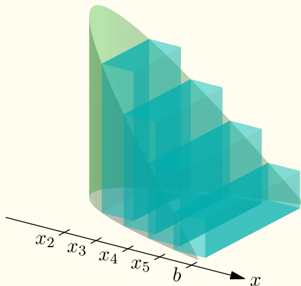
Figur 5.7: Volumet av geometrien (gul) tilnærmes ved summen av hver A(x_i)\Delta x (blå).
