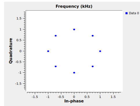
Figura 5. Diagrama de constelación 8-PSK obtenido a partir de la tabla de verdad.
