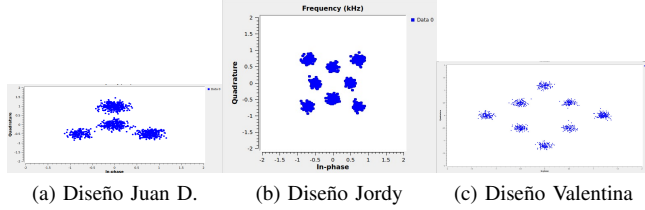
Figura 10. Dispersión de los símbolos para las constelaciones propuestas bajo canal AWGN.
