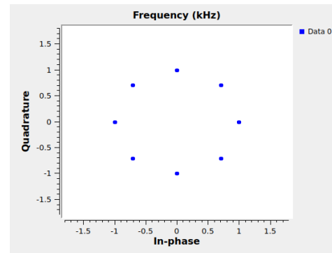
Figura 5. Diagrama de constelación 8-PSK obtenido a partir de la tabla de verdad.
