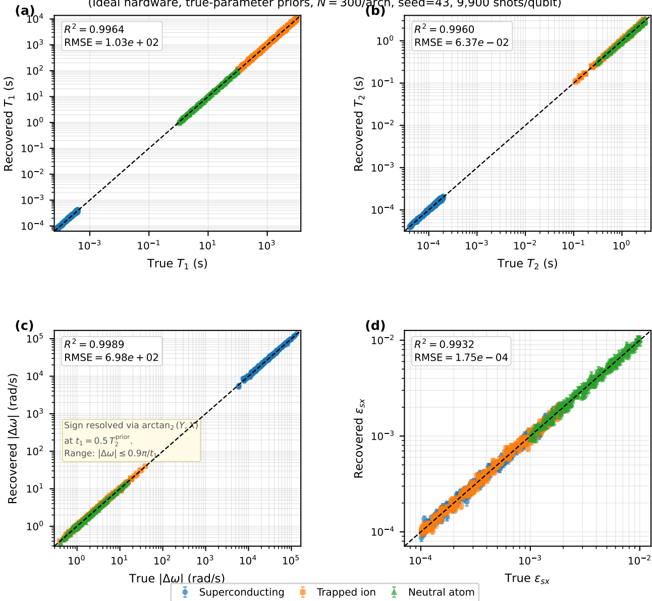
Fig. 2 — Parameter Recovery Accuracy
