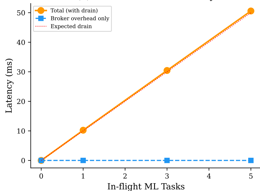
(d) GPU Reallocation Latency
