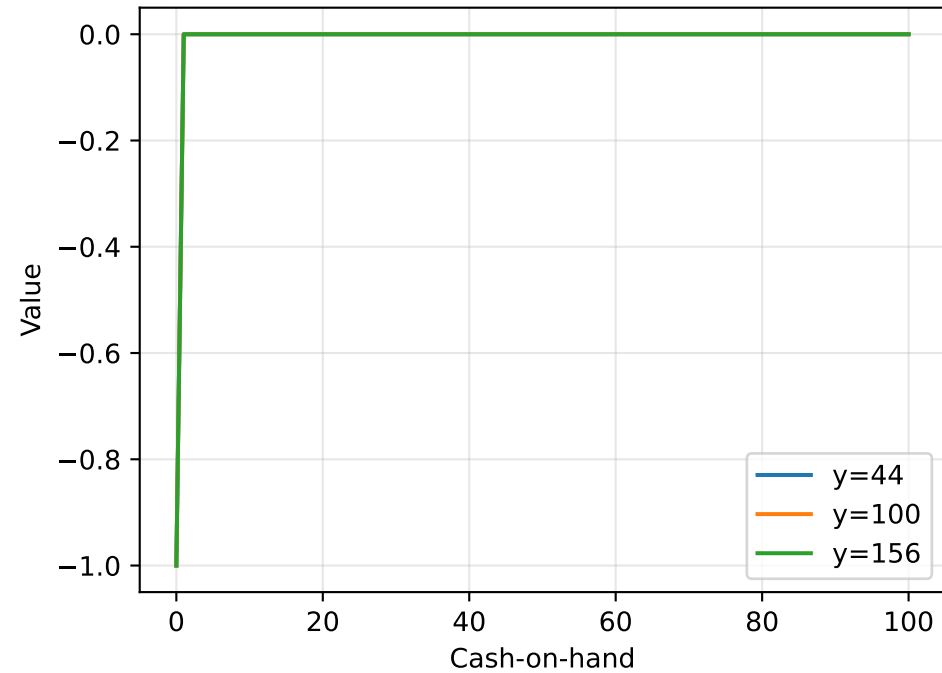
Value Function
