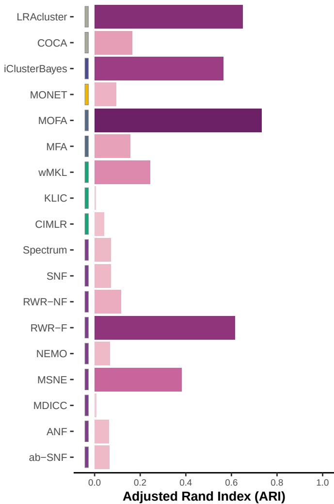
ARI bar chart: MOVICS
