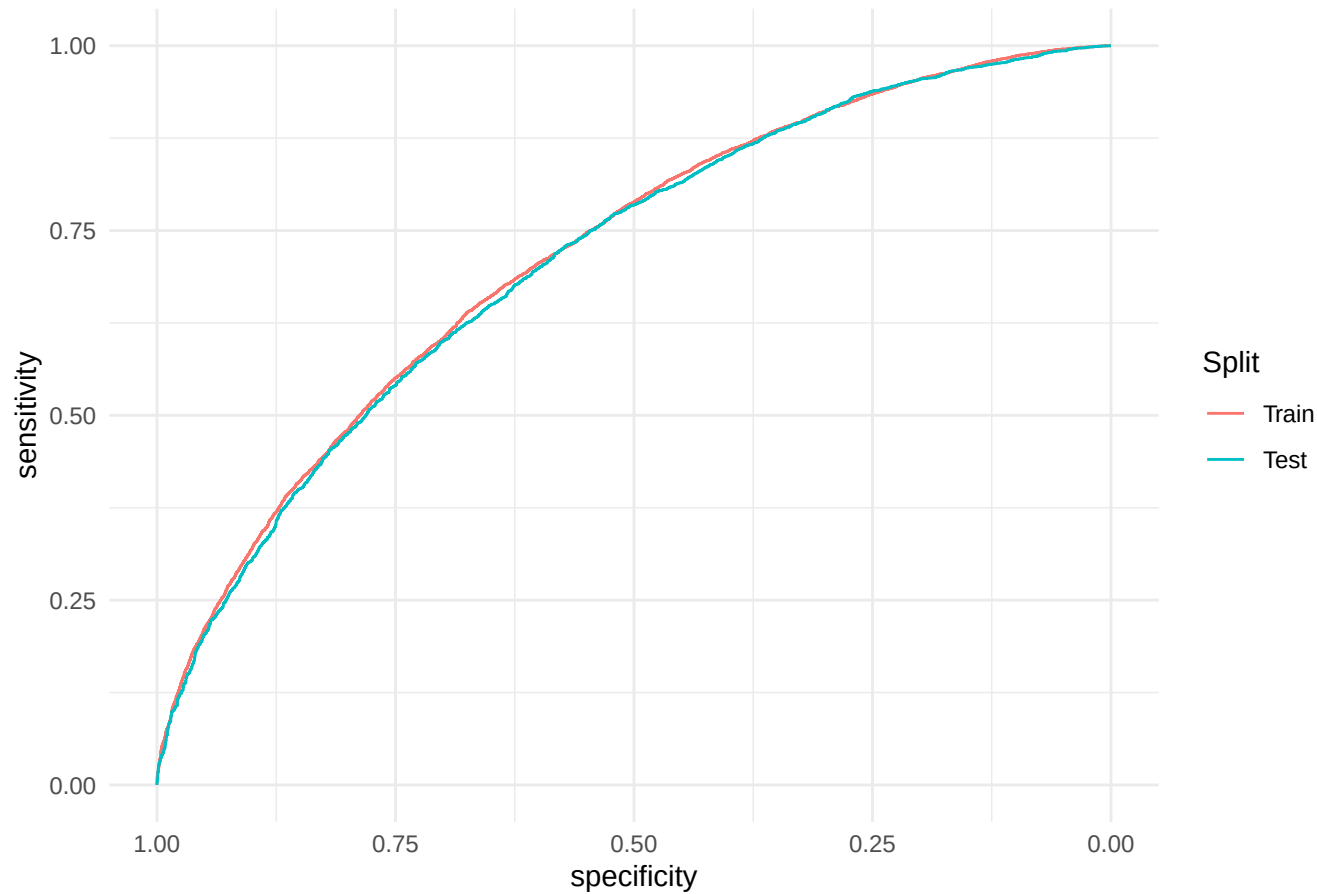
ROC — Train (AUC=0.717) vs. Test (AUC=0.712)
