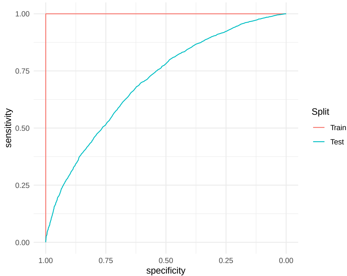
ROC – Train (AUC=1.000) vs. Test (AUC=0.705)
