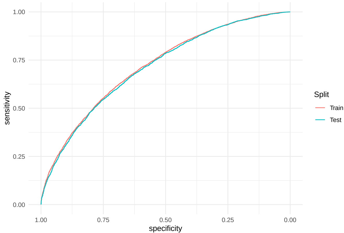
ROC — Train (AUC=0.718) vs. Test (AUC=0.712)
