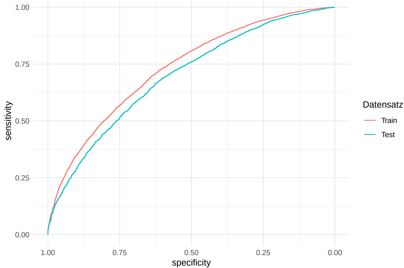
ROC Neuronales Netz — Train (AUC=0.732) vs. Test (AUC=0.696)
