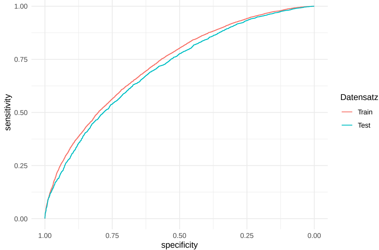
ROC Neuronales Netz — Train (AUC=0.728) vs. Test (AUC=0.708)
